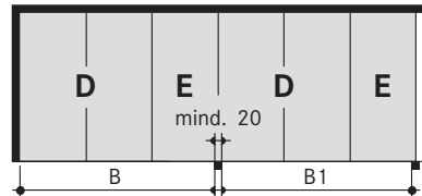
Kombinationsanlage (6 Pkw)
