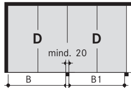
Doppelanlage (4 Pkw)
