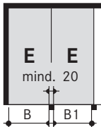
Einzelanlage (2 Pkw)
