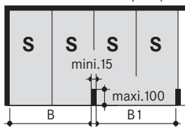
Deux installations simples (4 voitures)
