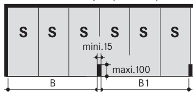
Trois installations simples (6 voitures)
