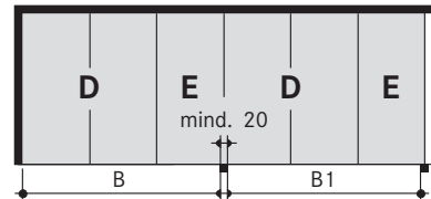
Kombinationsanlage (9 Pkw)
